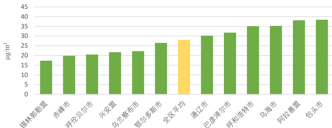
图2 12盟市细颗粒物 (PM 2.5 ) 浓度情况
